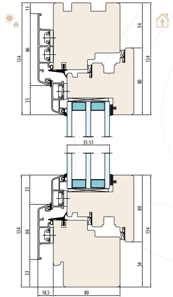
SYSTEM NATURO 80 ALU GEMINI CLASSIC Äußere Fensterbankkrügung
