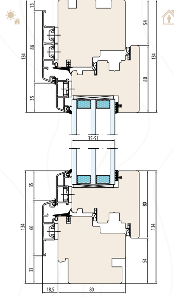
SYSTEM NATURO 80 ALU GEMINI CLASSIC Innen- und Außenfensterbankkrügung
