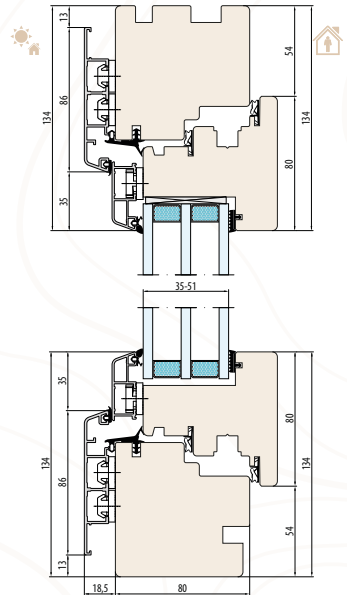
SYSTEM NATURO 80 ALU GEMINI CLASSIC Innere Fensterbankkrügung
