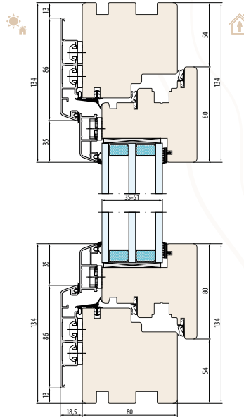
SYSTEM NATURO 80 ALU GEMINI CLASSIC Ohne Fensterbankkrügung
